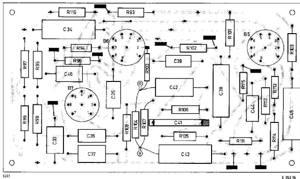
Fig. 32. Gedrukte-bedringsplaat E, ijkspanningsdeel
