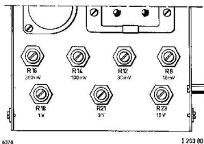
Fig. 5 Afregeling van de meetgebieden
