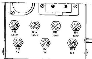
Fig. 16. Afregeling van de meetgebieden
