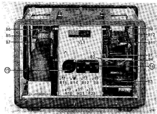
Fig. 23. Achteraanzicht
