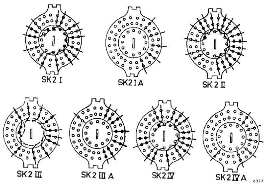
Fig. 34. Schakelaarsegmenten SK 2
