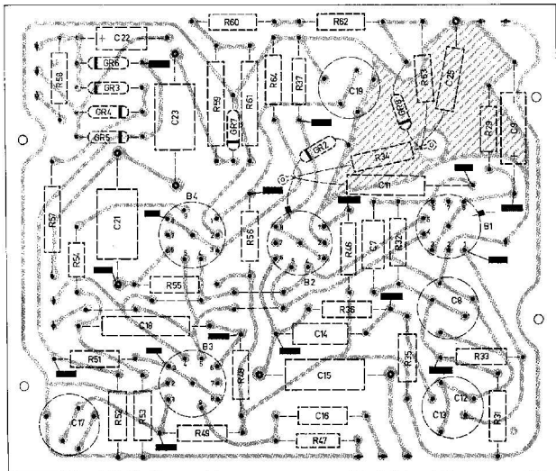
Fig. 29. Gedrukte-bedradingsplaat A, versterker (bedrading)
