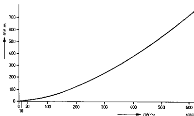
Fig. 9. Diodekarakteristiek
