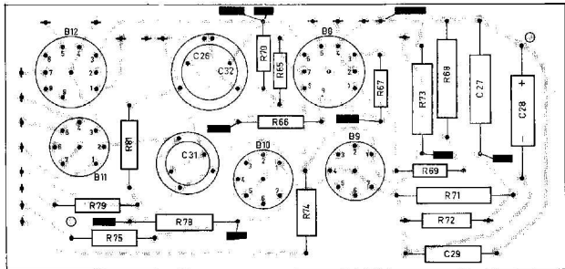
Fig. 31. Gedrukte-bedragsplaat D, voedingsdel
