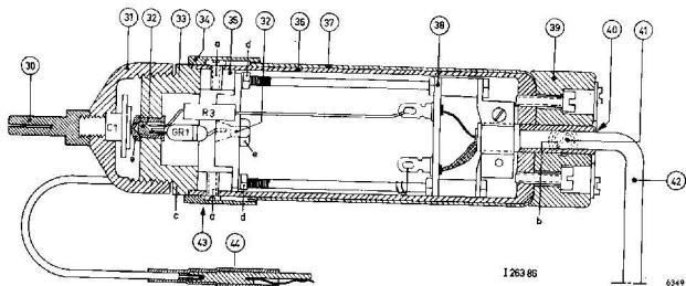
Fig. 35. Meetekop
