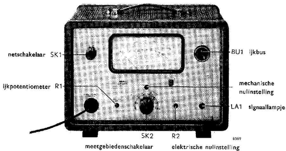
Fig. 4. Vooraanzicht
