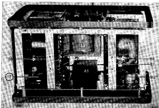
Fig. 24. Bovenaanzicht
