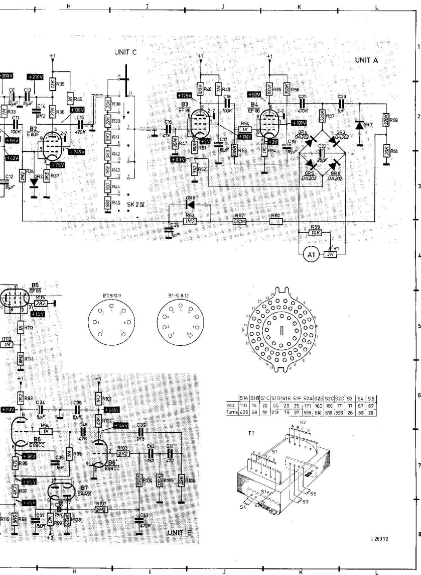
36. Schema GM 6025 - Fig. 36 Schéma GM 6025
