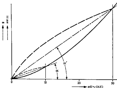
Fig. 10. Versterkerkarakteristiek
