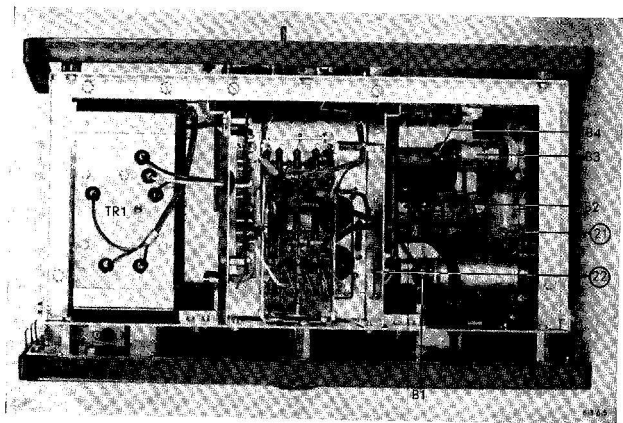
Fig. 26. Onderaanzicht
