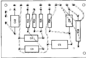
Fig. 30. Gedrukte-bedragsplaat B, filter
