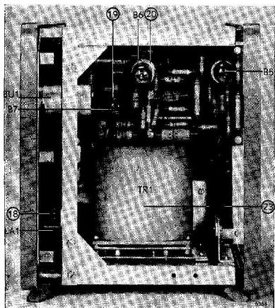
Fig. 24. Bovenaanzicht
