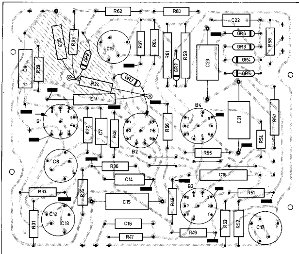
Fig. 28. Gedrukte-bedradingsplaat A, versterker (onderdelen)
