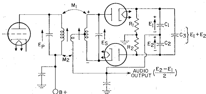
Fig. 33—Ratio-detector circuit.
