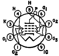
SQL
