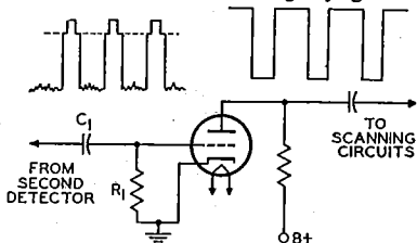
Fig. 80—Sync-separator circuit.
