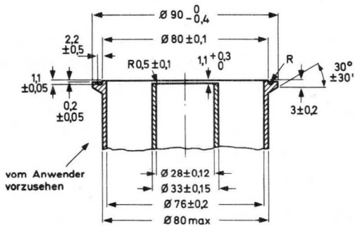
Koaxialleitung 76/33 7259894V2
