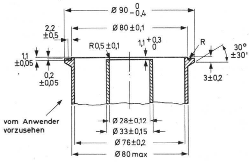
Koaxialleitung 76/33 7Z59894V2
