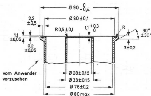
Koaxialleitung 76/33 7259894V2
