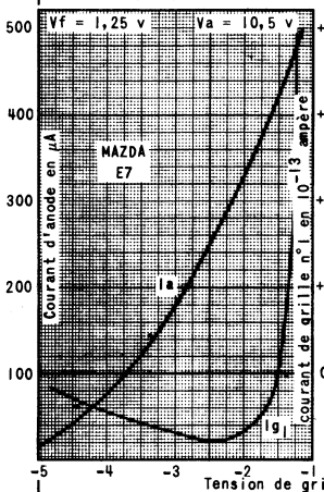
Courbes du courant d'anode et du courant de grille n° 1 en fonction de la tension de la grille n° 1 MONTAGE TRIODE
